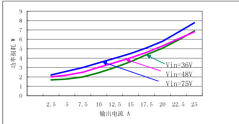
输出电流与损耗关系曲线
