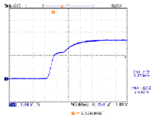
输出上升时间
