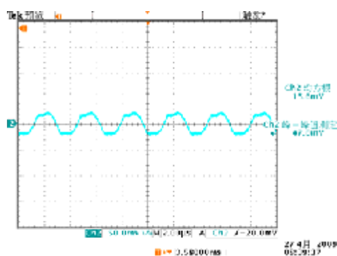
输出纹波
